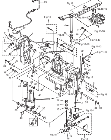
Fig. 20 BRACKET (POWER TRIM & TILT) ブラケット (パワートリム & チルト)
